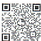
QR Code
